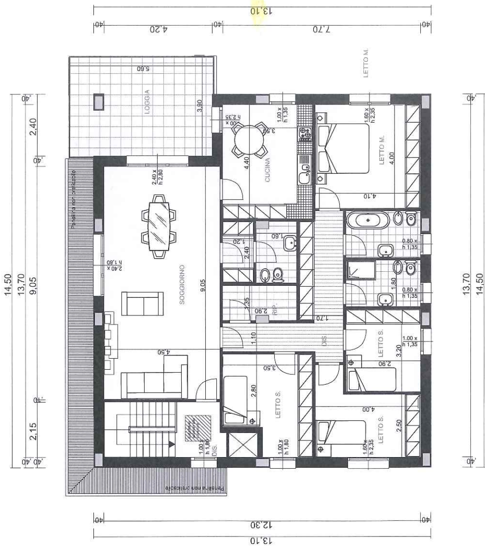
Pianta primo piano - Soluzione 4 camere H. min. 3.20 H.max 4.40
